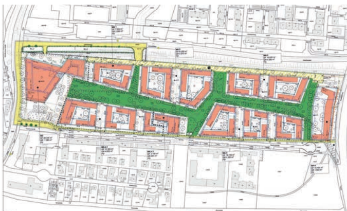
Planzeichnung vom Neuen Mitterfeld (Stand: Juli 2023). Bild: bgsm
